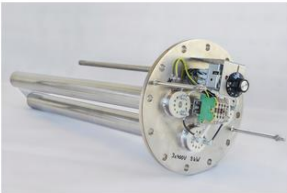
Boilerflansch mit 3 Rohren
